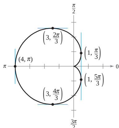
Rectas tangentes horizontales y verticales de r = 2(1 - \cos \theta)
