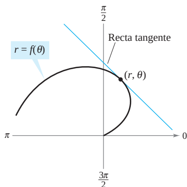
Recta tangente a una curva polar
