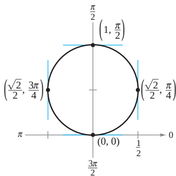
Rectas tangentes horizontales y verticales a r = \sin \theta
